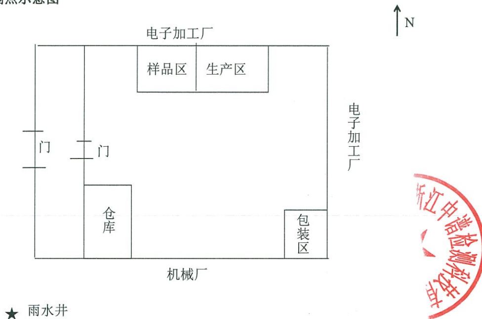
雨水测点示意图
